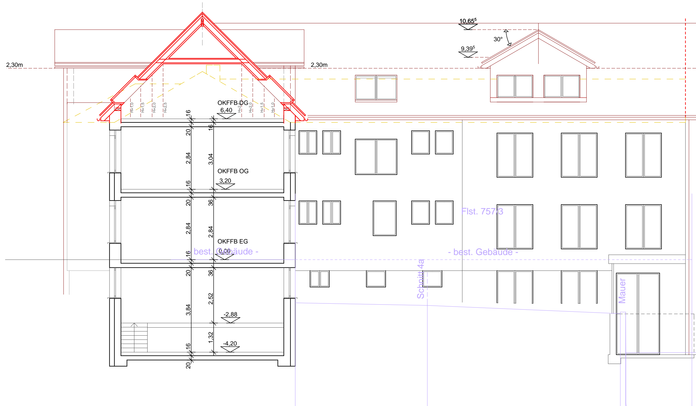
Ansicht OST,A-A_m.1.100_20.03.2014
