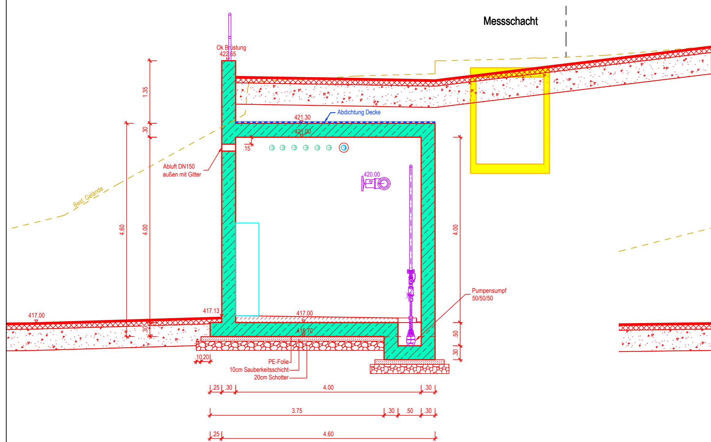
Schnitt A-A
