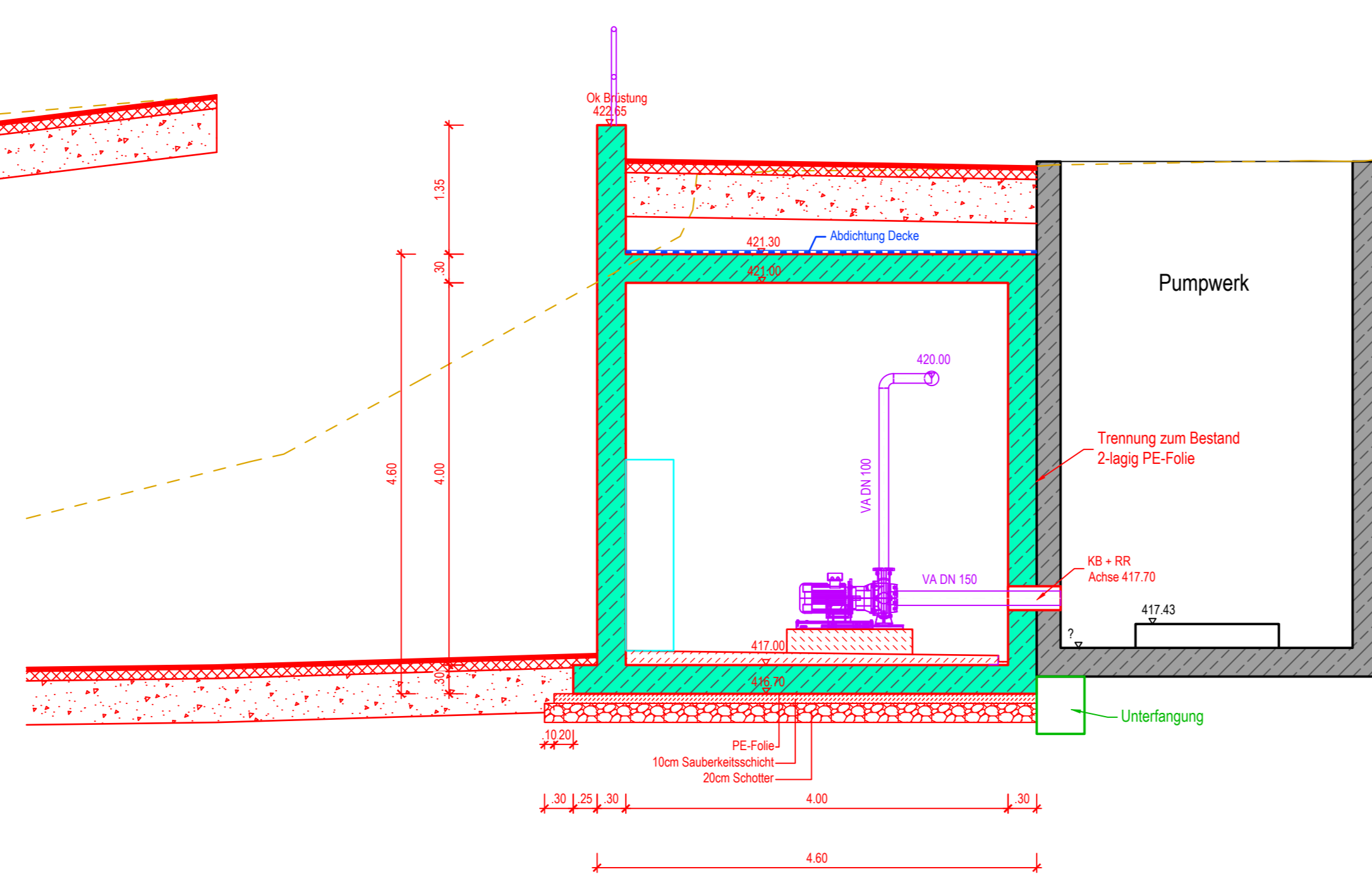
Schnitt B-B
