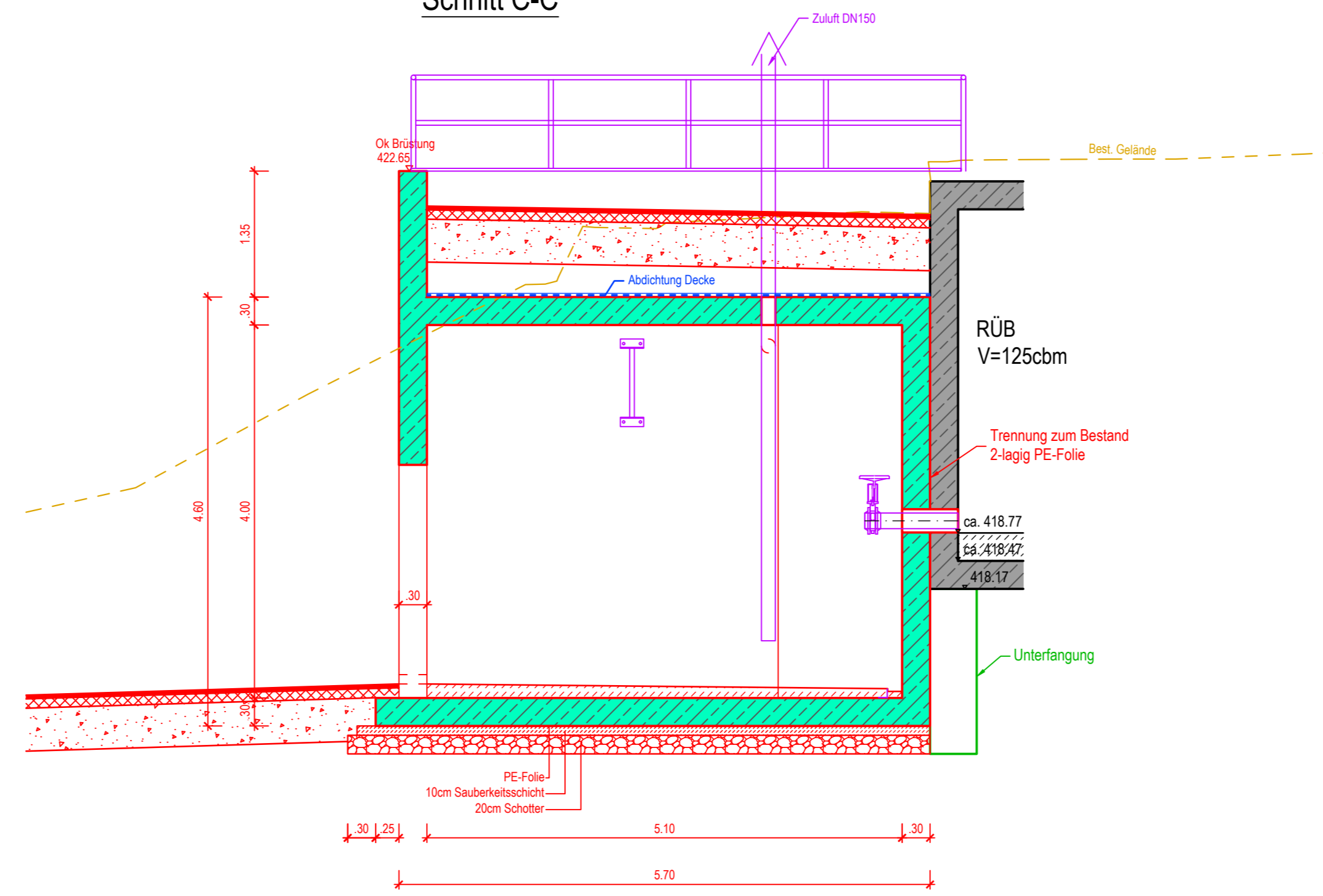
Schnitt C-C
