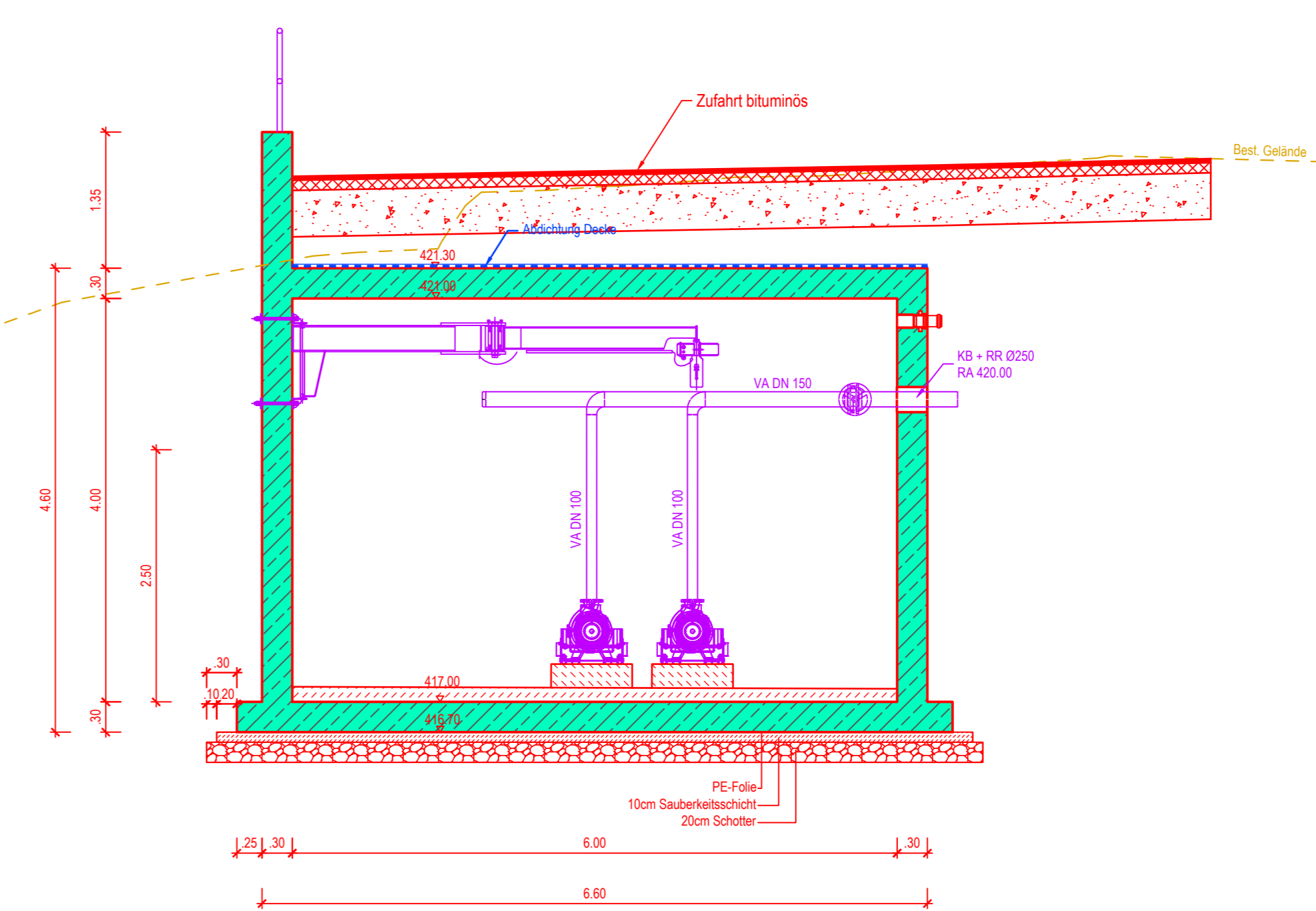
Schnitt 1-1
