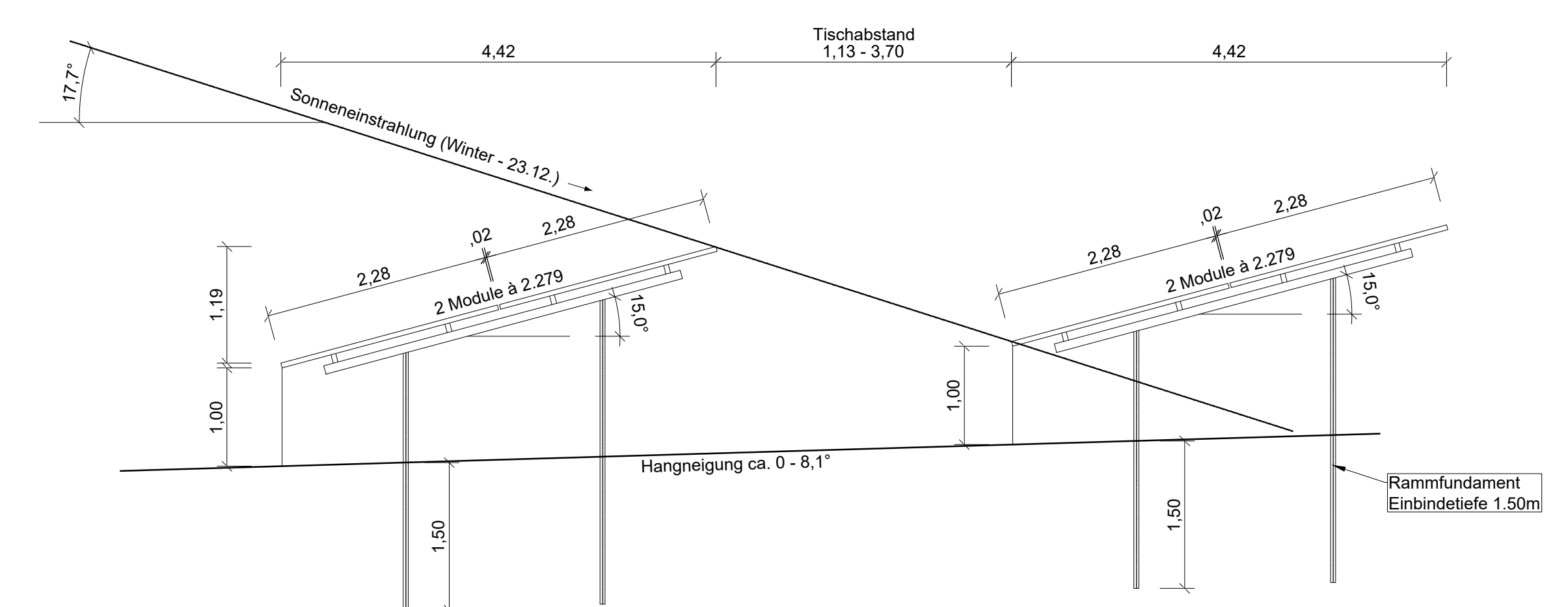
Querschnitt M 1:50
